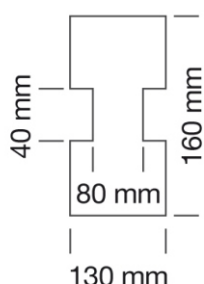
Sezione Palo
