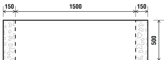
ANELLO PROLUNGA 150 x 150 H. 50
