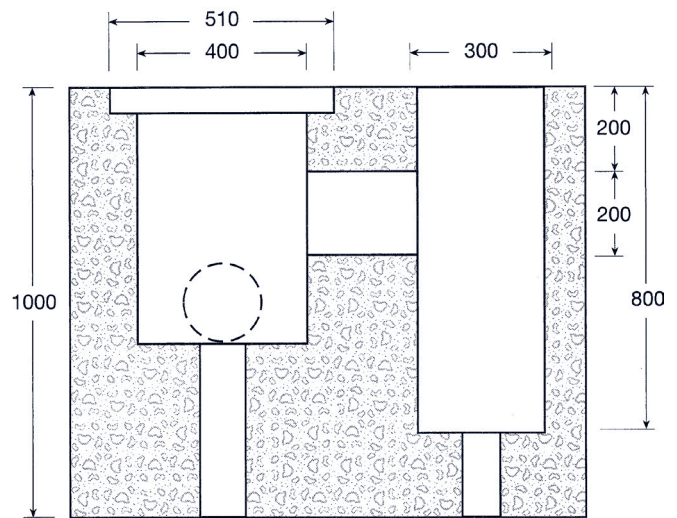
SEZ. A
