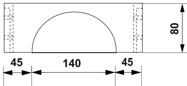
ANELLO PROLUNGA 200X200 H. 80
