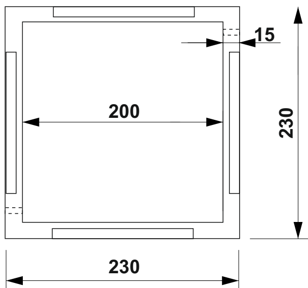
PIANTA
