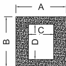
FORO 50x70 (SOLO SU ORDINAZIONE)
