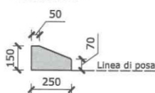
C3 VISTA LATERALE SPARTITRAFFICO "LOMBARDA" Testata a 90°
