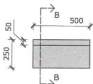
C2 SEZIONE B-B SPARTITRAFFICO "LOMBARDA" L=50 cm
