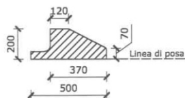
C1 SEZIONE A-A SPARTITRAFFICO "PROVINCIA" L=50 cm
