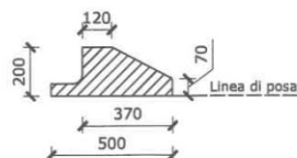
C3 SEZIONE C-C SPARTITRAFFICO "PROVINCIA" Testata a 90°
