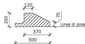
C2 SEZIONE B-B SPARTITRAFFICO "PROVINCIA" L=30 cm
