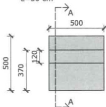
C1 SEZIONE A-A SPARTITRAFFICO "PROVINCIA" L=50 cm
